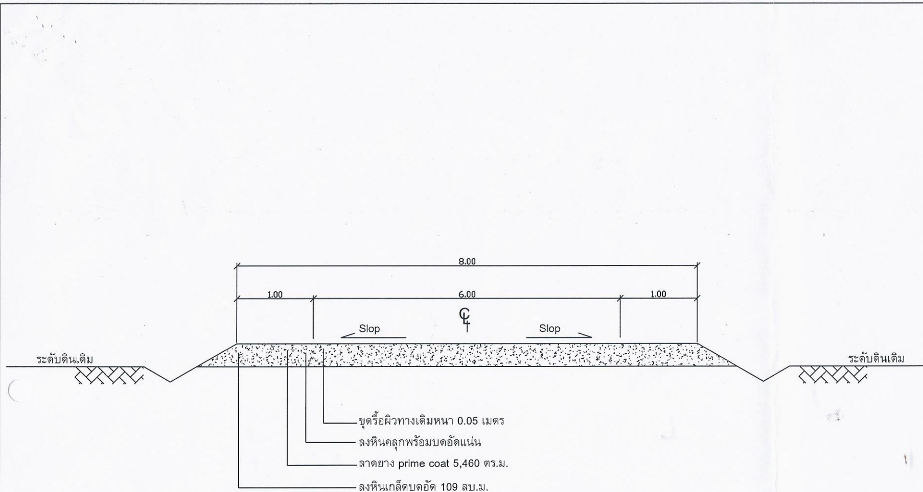
รูปตัดถนนลาดยาง
